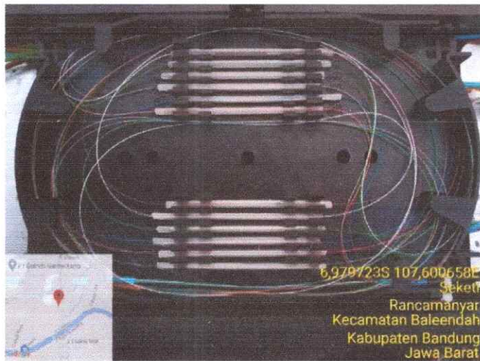
ODP SGY 014 OUTPUT SPLITTER
