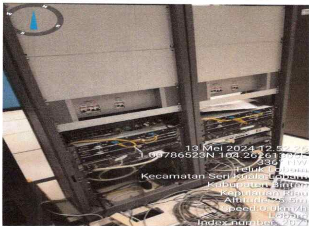
IDU LOBAM
