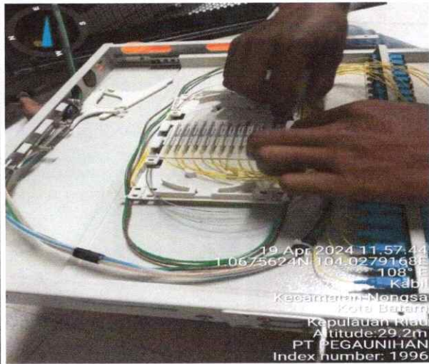
Pemasangan core di otb
