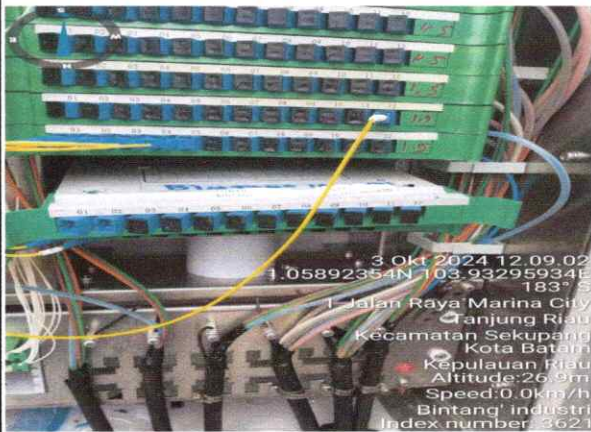
ODC SIMPANG POLSEK BATU AJI
