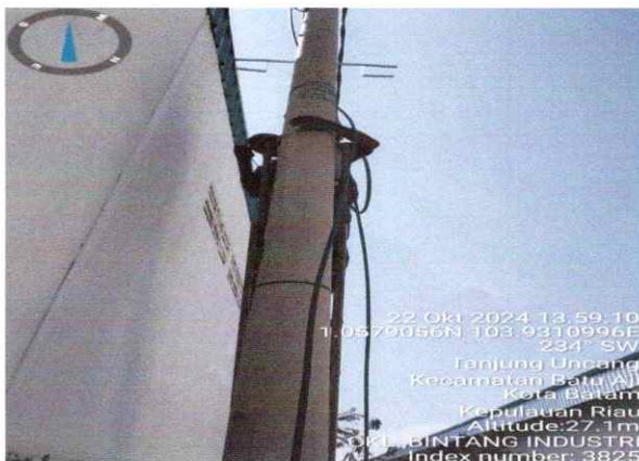
PEMASANGAN AKSESORIES TIANG
