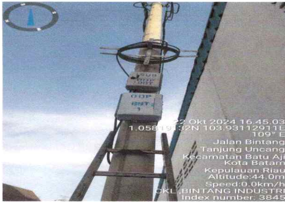
PEMASANGAN ODP
